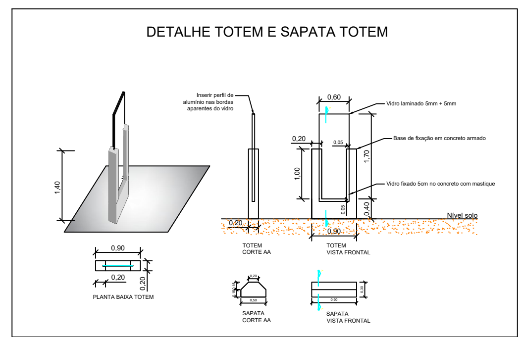
DETALHE TOTEM E SAPATA TOTEM
