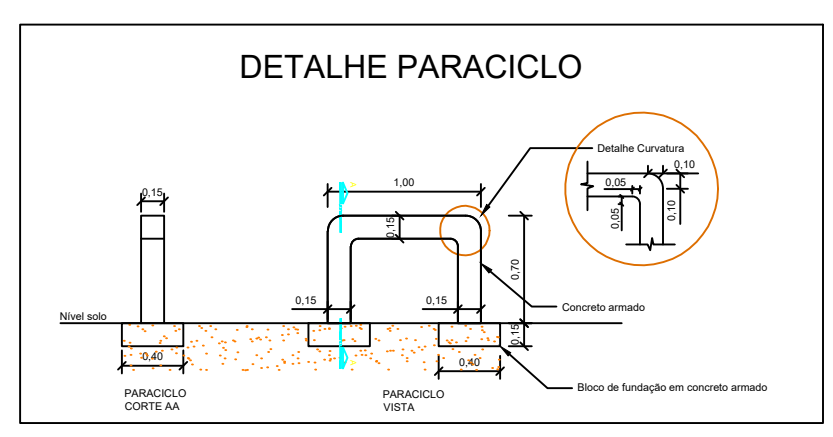
DETALHE PARACICLO
