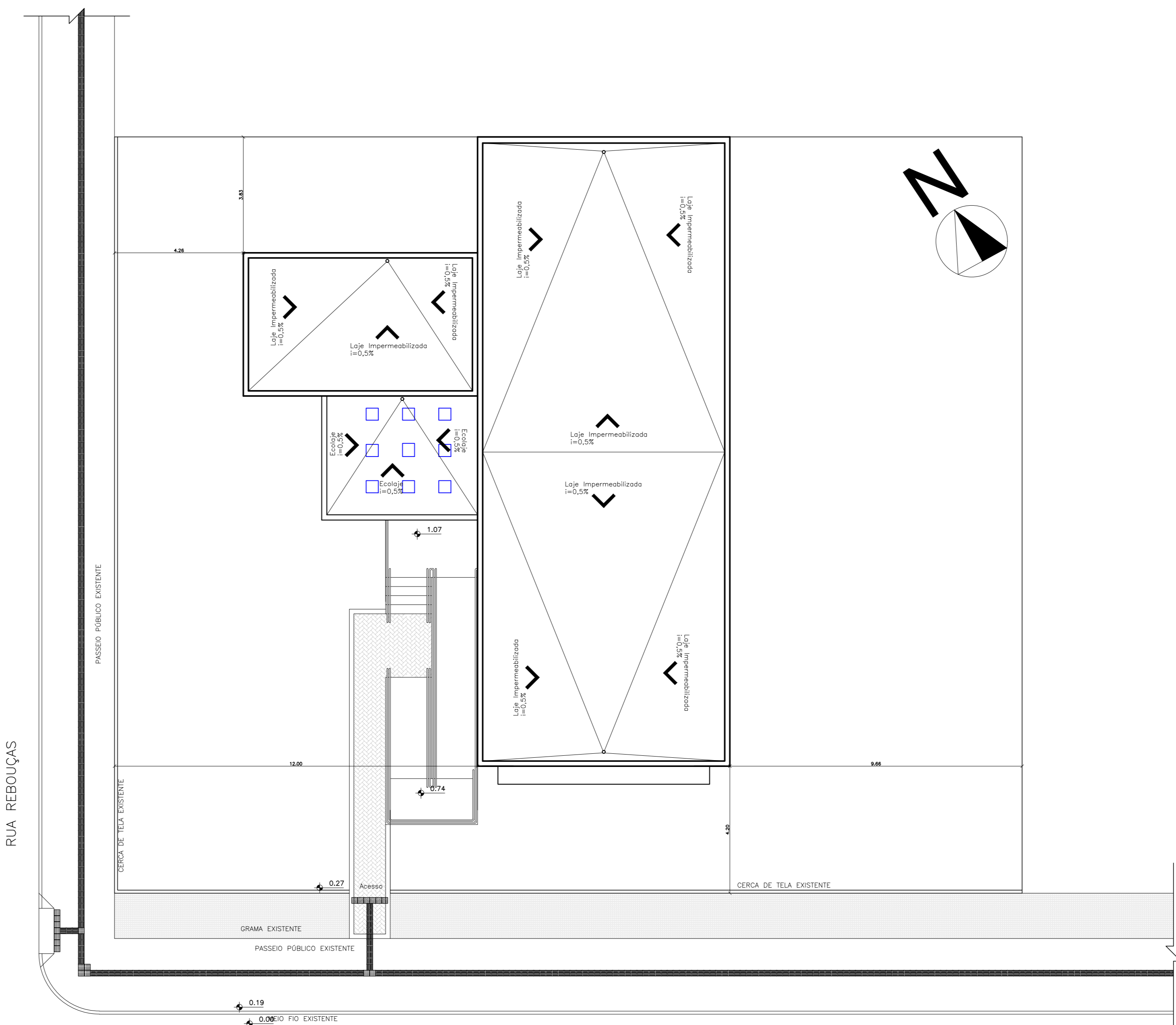
Planta de Cobertura esc 1:100
