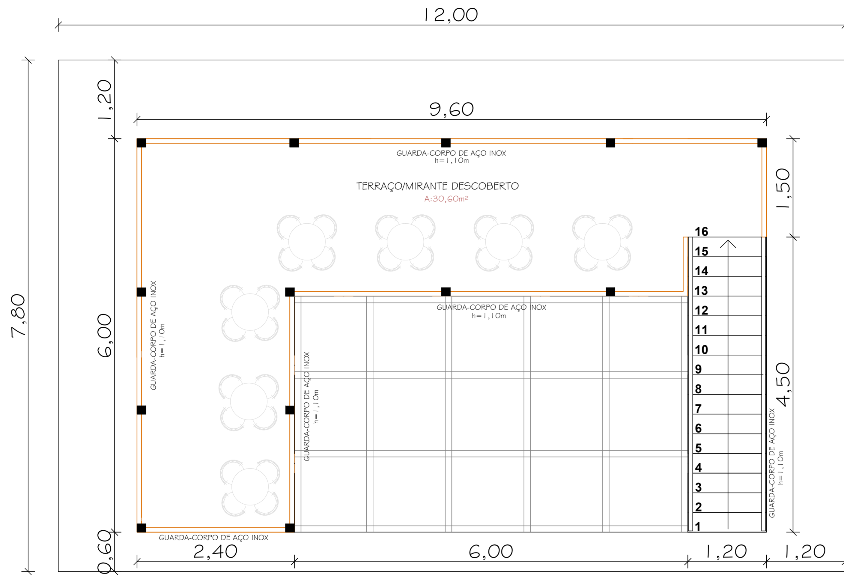
Planta Baixa - Superior Quiosque container
