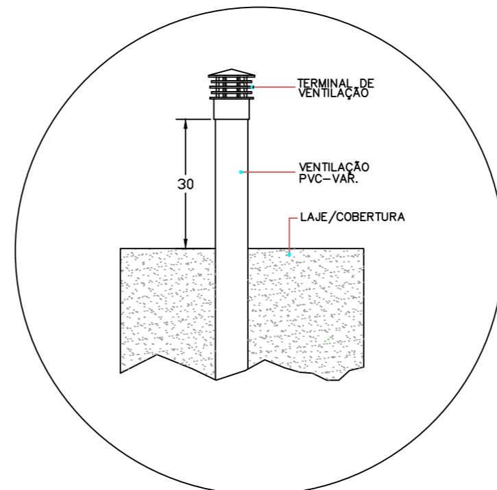
DETALHE SAÍDA DA VENTILAÇÃO SEM ESCALA
