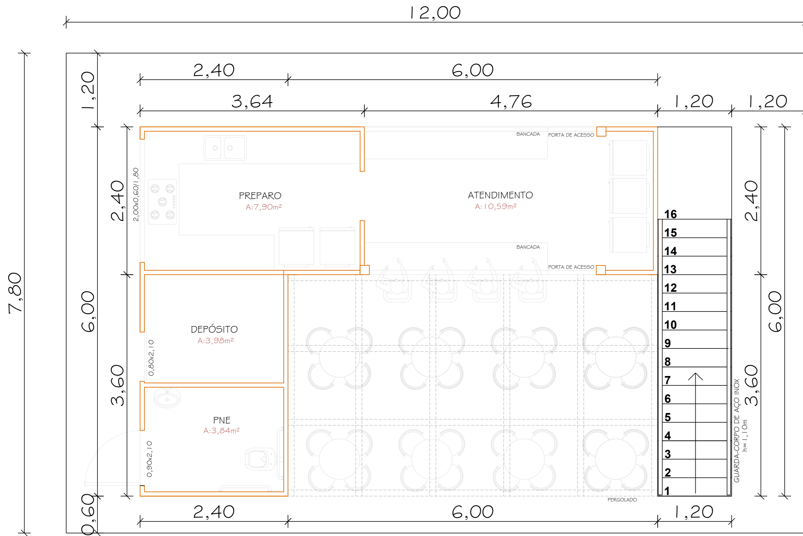
Planta Baixa - Quiosque container AT: 50,60 m² ESC: 1/50
